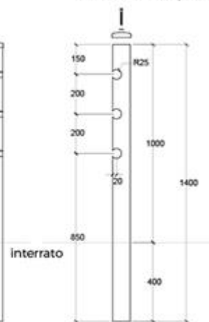
vista laterale / esploso
